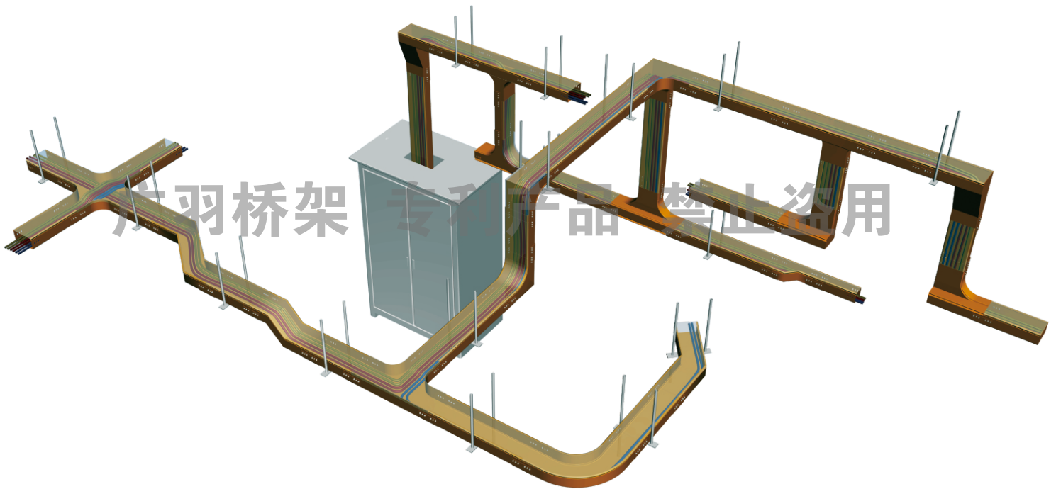
Cable trunking Layout Diagram 電綫槽空間布置示意圖 ▲
